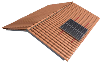
Perfiles paralelos a la cumbrera
