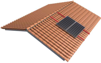
Perfiles perpendiculares a la cumbrera
