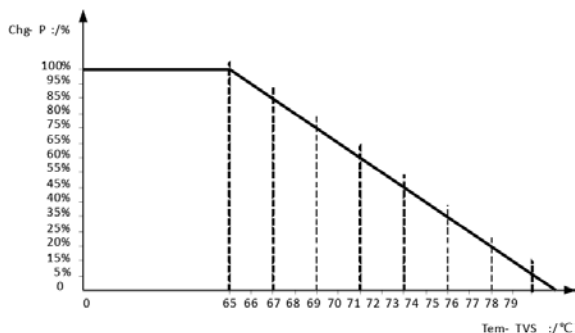
Figura 8. Gráfico de protección de sobrecalentamiento
