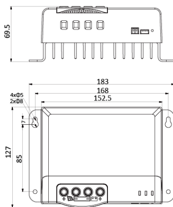
Modelo: MC2450N10 Dimensiones del contorno: 183*127*69.5mm Dimensiones del montaje: 168*85mm Diámetro agujeros: Φ5mm Especificaciones del cable: 20-6AWG
