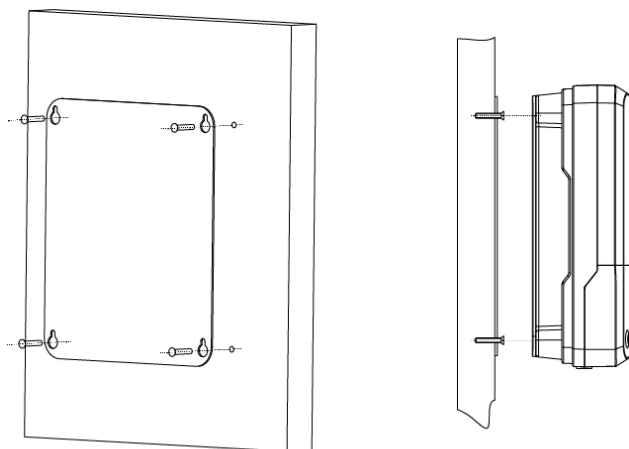
Fig 6. Fije el regulador solar
