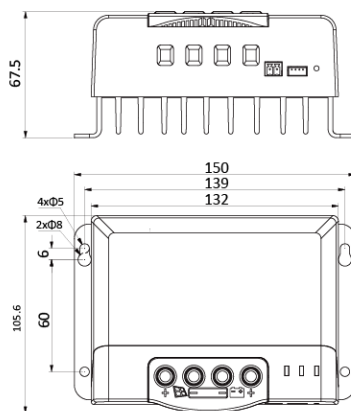
Modelo: MC2430N10 Dimensiones del contorno: 150*105.6*67.5mm Dimensiones del montaje: 139*60mm Diámetro agujeros: Φ5mm Especificaciones del cable: 20-6AWG
