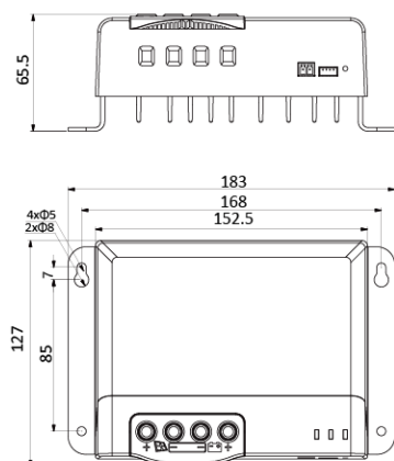
Modelo: MC2440N10 Dimensiones del contorno: 183*127*65.5mm Dimensiones del montaje: 168*85mm Diámetro agujeros: Φ5mm Especificaciones del cable: 20-6AWG
