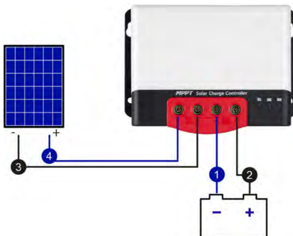
Fig 7. Cableado
