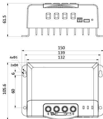
Modelo: MC2420N10 Dimensiones del contorno: 150*105.6*61.5mm Dimensiones del montaje: 139*60mm Diámetro agujeros: Φ5mm Especificaciones del cable: 20-6AWG
