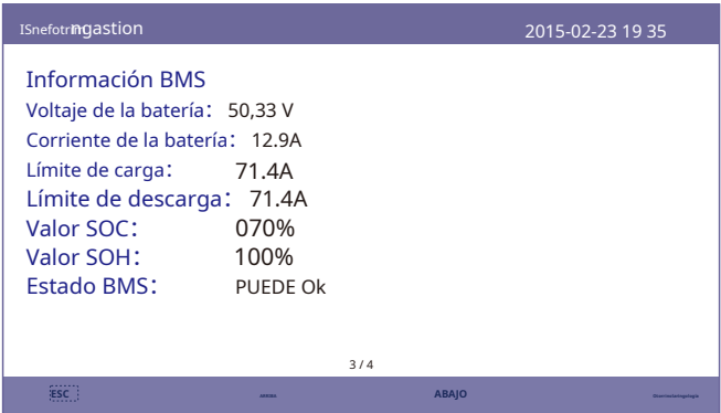
Figura 5.7 Página de información 3
