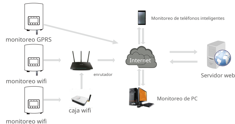
Figura 4.14 Función de comunicación Wi-Fi o GPRS
