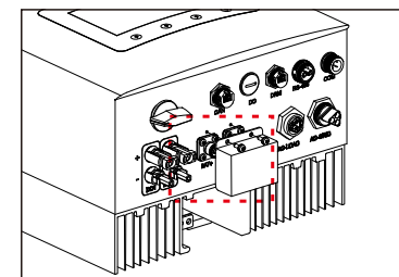
Figura 4.7 Instalación de la cubierta de protección de terminales
