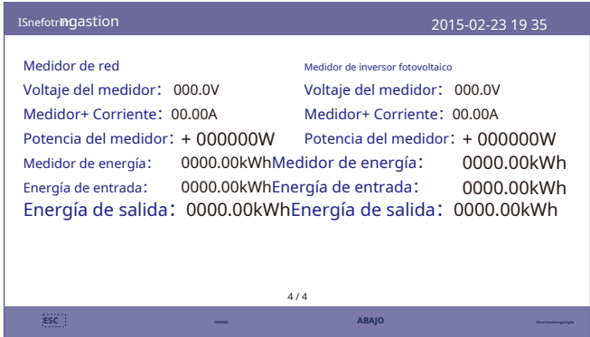
Figura 5.8 Página de información 4
