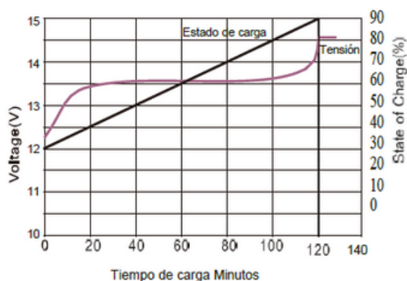
Curvas de estado de carga (0.5C, 25°C)
