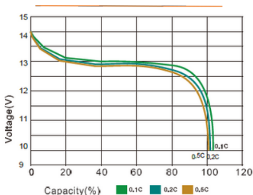
Curvas de estado de carga (0.5C, 25° C)
